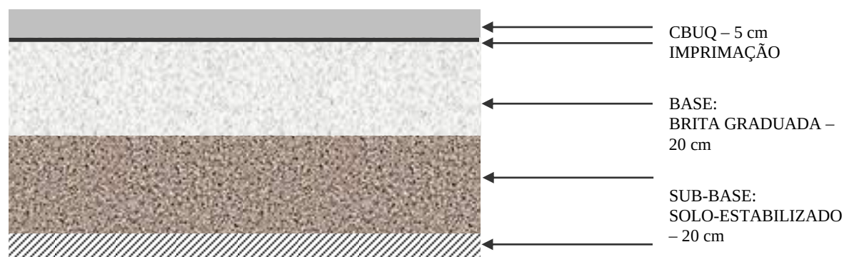
Figura 10 - Estrutura típica do pavimento
